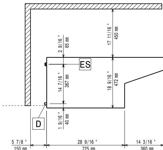
Felülnézet
